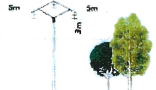
Sur isolateurs suspendus
